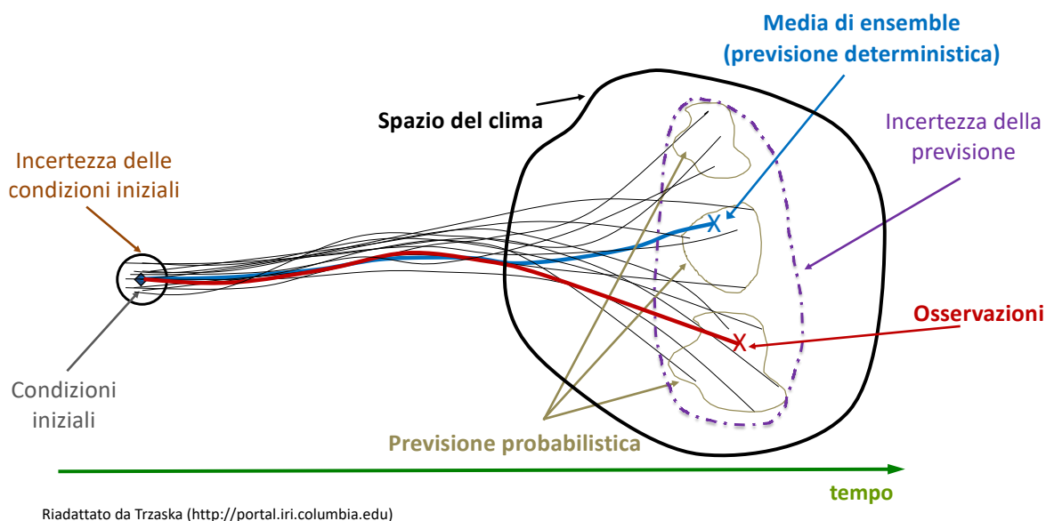
Figura 4.1: esempio schematico del processo di produzione di un "ensemble forecast". Lo schema illustra l'approccio che è normalmente utilizzato per produrre previsioni climatiche con modelli numerici del clima, a diverse scale temporali, da quelle sub-stagionali, alle previsioni stagionali e interannuali, fino alle decennali.
