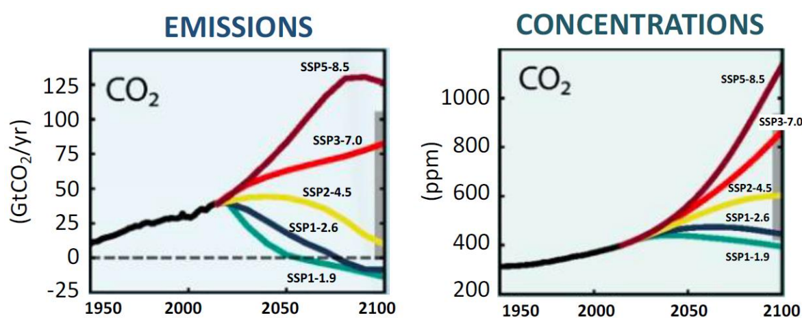
Figura 3.1: andamento delle emissioni (pannello a sinistra) e delle relative concentrazioni (pannello a destra) di gas a effetto serra, espresse in termini di CO 2 equivalente, ricostruite per il periodo storico (curva nera) e per i diversi scenari socioeconomici immaginati per il futuro (curve colorate). Le emissioni sono espresse in Giga-Tonnellate di CO 2 equivalente per anno e le concentrazioni in parti per milione (ppm). Fonte: IPCC-AR6, 2021.
