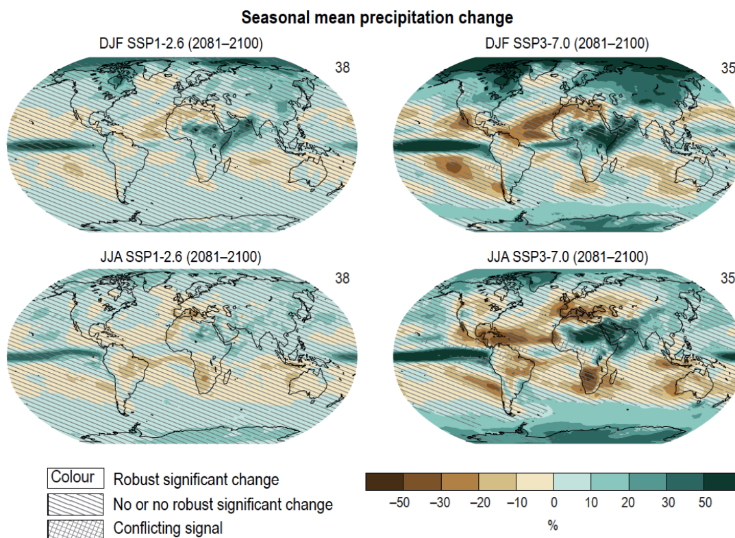
Figura 3.4: Variazione a lungo termine (esprese in %) delle precipitazioni medie stagionali, ottenute come medie di un ensemble multi-modello di proiezioni, per la stagione dicembre-gennaio-febbraio (DJF, pannelli in alto) e giugno-luglio-agosto (JJA, pannelli in basso). La differenza è calcolata tra le precipitazioni stagionali medie nel periodo 2081–2100 rispetto al periodo di riferimento 1995–2014, per (pannelli a sinistra) lo scenario SSP1–2.6 e (pannelli a destra) lo scenario SSP3–7.0. Il numero di modelli utilizzati è indicato in alto a destra nelle mappe. Le linee diagonali indicano le regioni dove i cambiamenti non sono significativi o dove meno del 66% dei modelli mostra cambiamenti superiori alla soglia di variabilità interna. Ulteriori dettagli sulle fonti e sull'elaborazione dei dati IPCC–AR6 (2021), Tabella 4.SM.1.
