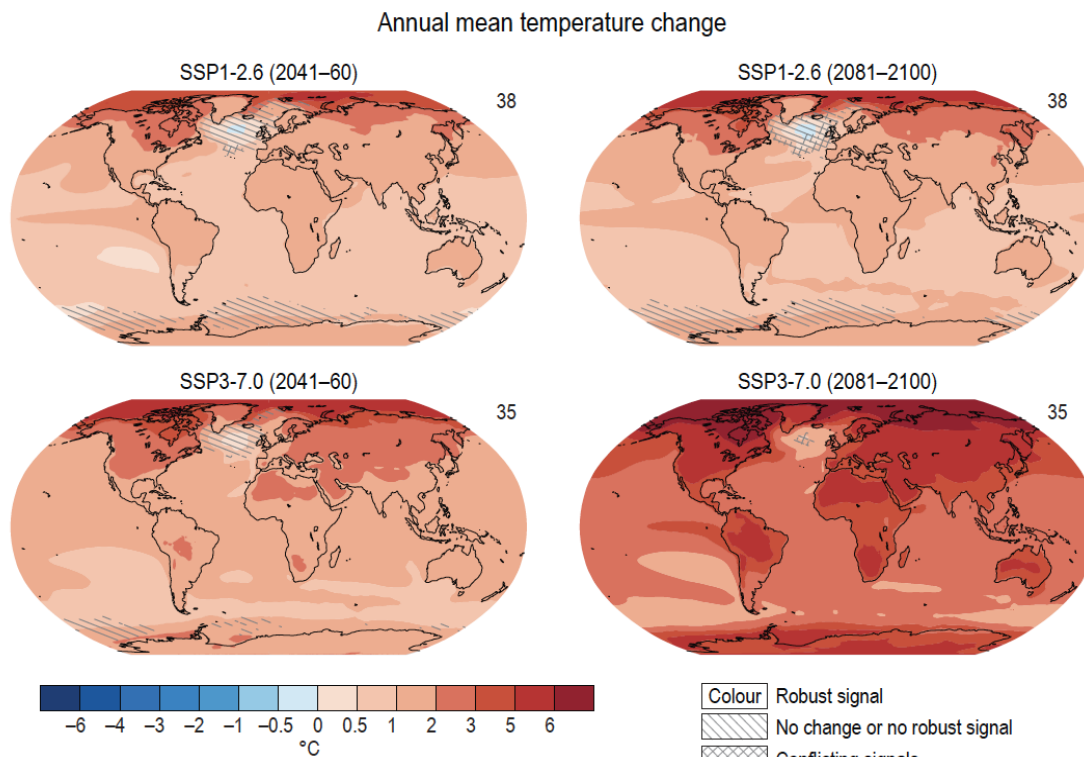
Figura 3.3: Variazioni della media annuale della temperatura superficiale (°C), ottenute come medie di un ensemble multi-modello di proiezioni, per i periodi 2041–2060 e 2081–2100, rispetto al periodo di riferimento 1995–2014. Pannelli in alto scenario SSP1–2.6 e in basso scenario SSP3–7.0. Il numero di modelli utilizzati è indicato in alto a destra nelle mappe. Le linee diagonali indicano regioni senza cambiamenti significativi.
