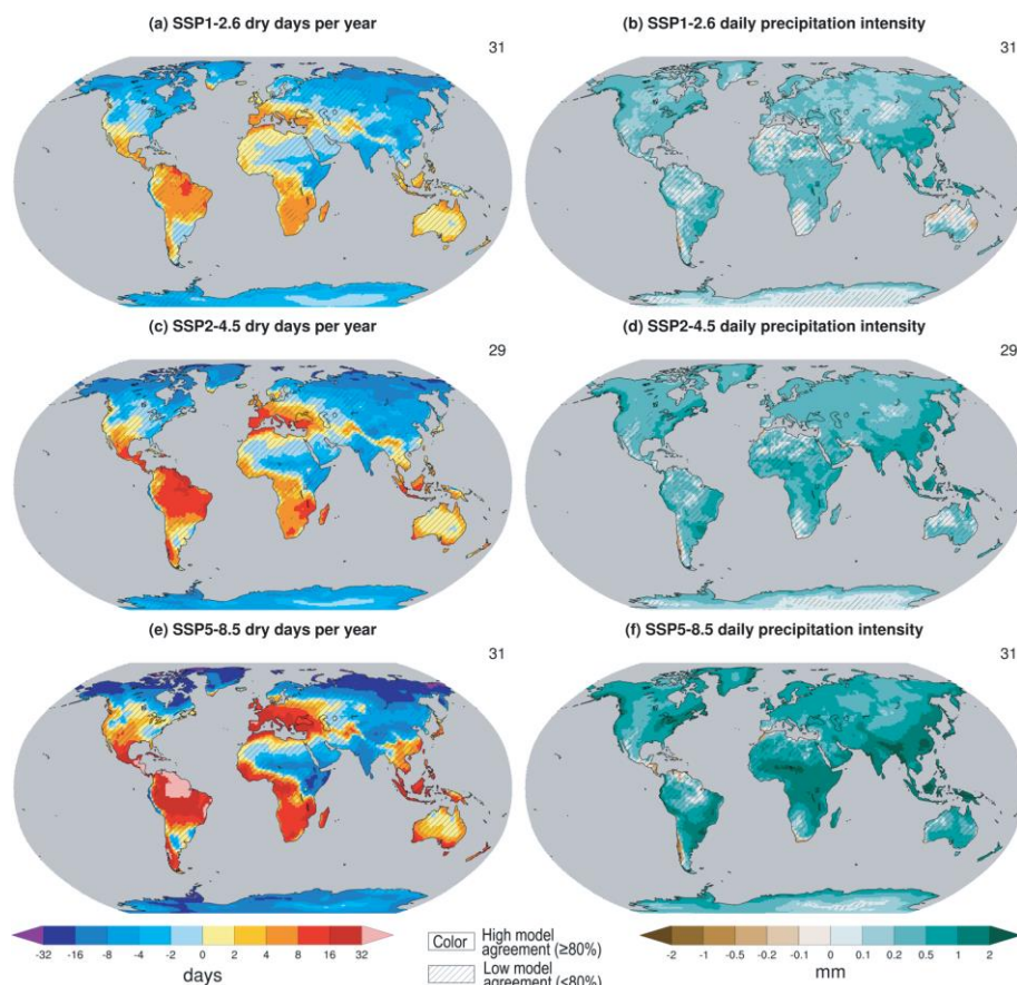
Figura 3.5: Variazioni nelle statistiche sulle precipitazioni giornaliere proiettate a lungo termine in tre futuri scenari di emissioni. Pannelli a sinistra: cambiamento delle medie annuali nel numero di giorni asciutti (ovvero giorni con meno di 1 mm di pioggia); pannelli a destra: cambiamento delle medie annuali nell'intensità giornaliera delle precipitazioni (in mm, stimata come quantità media giornaliera di precipitazioni nei giorni piovosi – ad esempio, giorni con intensità superiore a 1 mm/giorno) calcolata in media tra i modelli CMIP6 disponibili (numero fornito in alto a destra di ogni pannello). Pannelli a) e b) scenario SSP1-2.6; pannelli c) e d) scenario SSP2-4.5; pannelli e) ed f) scenario SSP5-8.5. Le linee diagonali indicano aree dove meno dell'80% dei modelli concorda sul segno del cambiamento. Ulteriori dettagli sulle fonti e sull'elaborazione dei dati sono disponibili in IPCC-AR6 (2021), Tabella 8.SM.1.
